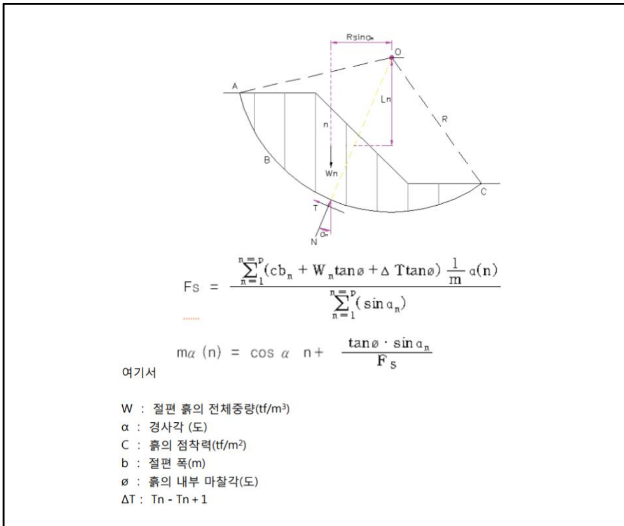
【그림 8.7】 Bishop의 안전율 계산식
