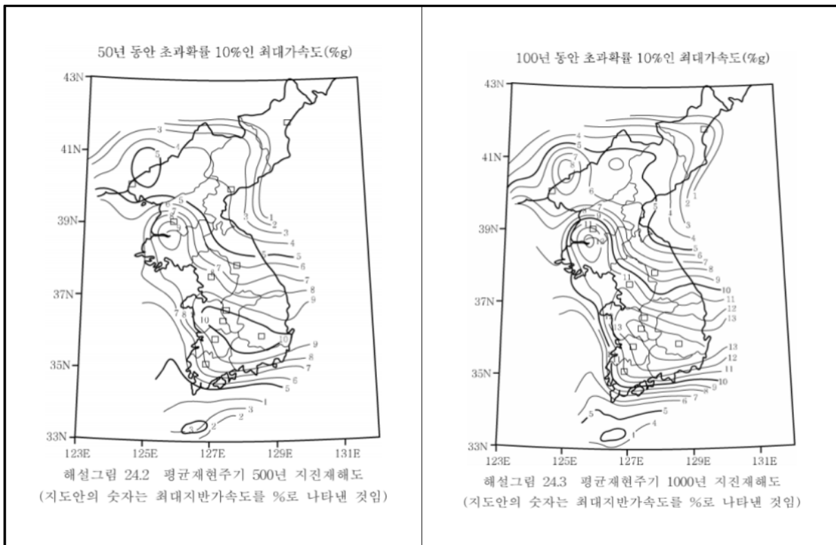
【그림 8.12】 평균재현주기 500년 및 1000년 지진재해도
