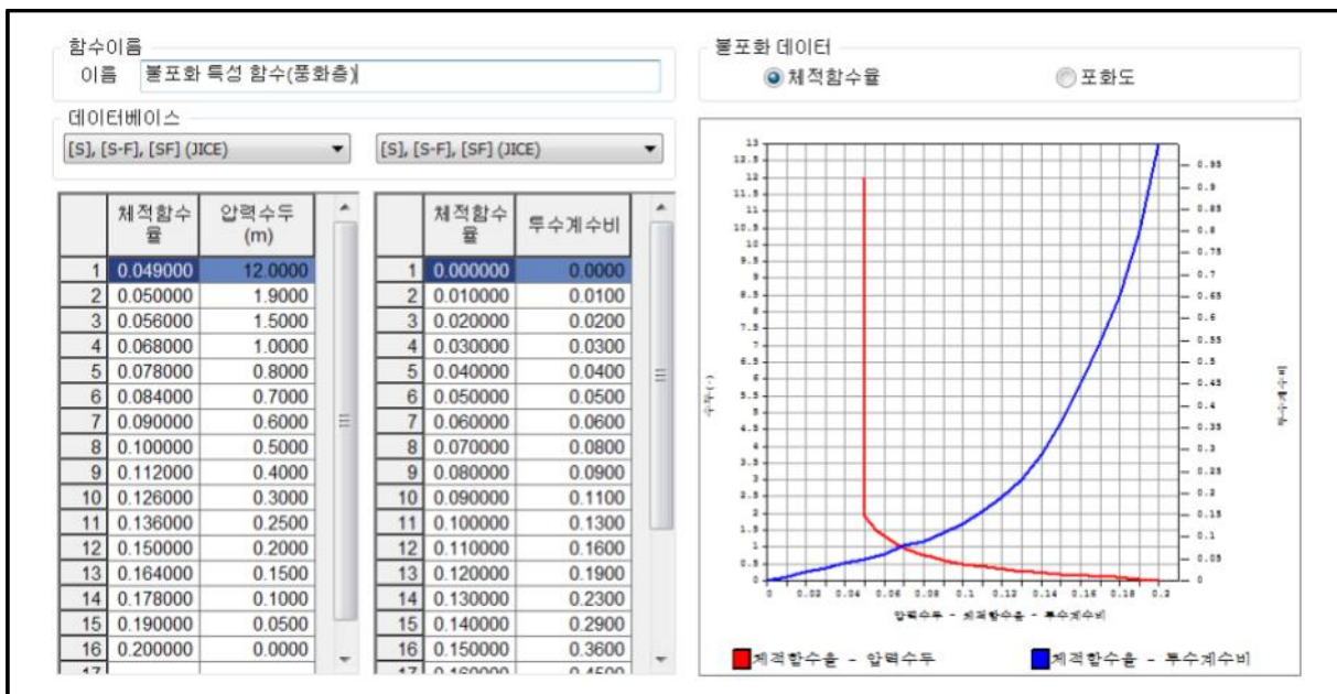
【그림 8.14】 압력수두-채적함수(포화도)-투수계수비 함수
