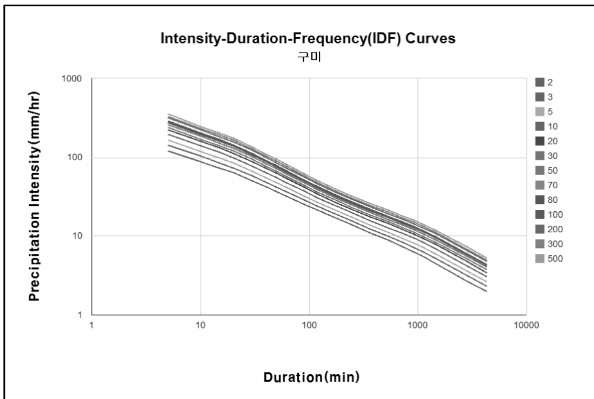
【그림 8.9】 구미지역 IDF곡선
