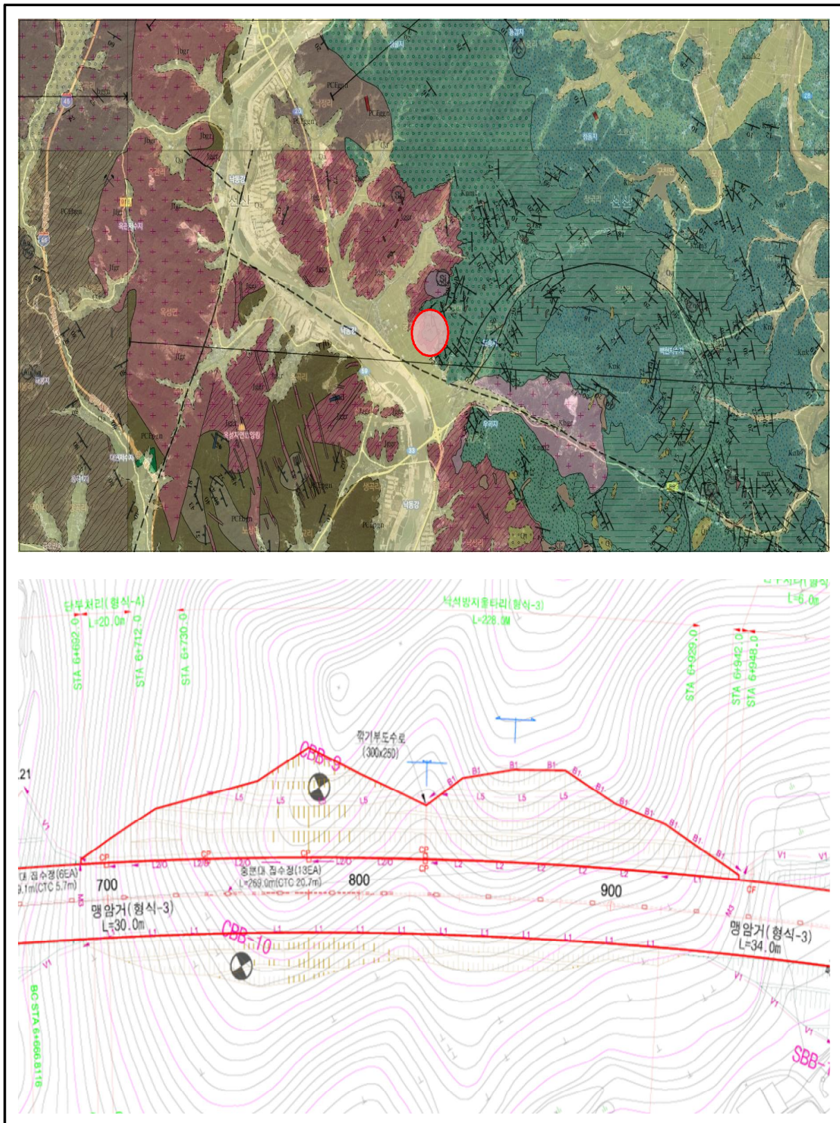
【그림 8.13】 상주절토08 검토대상 비탈면구간
